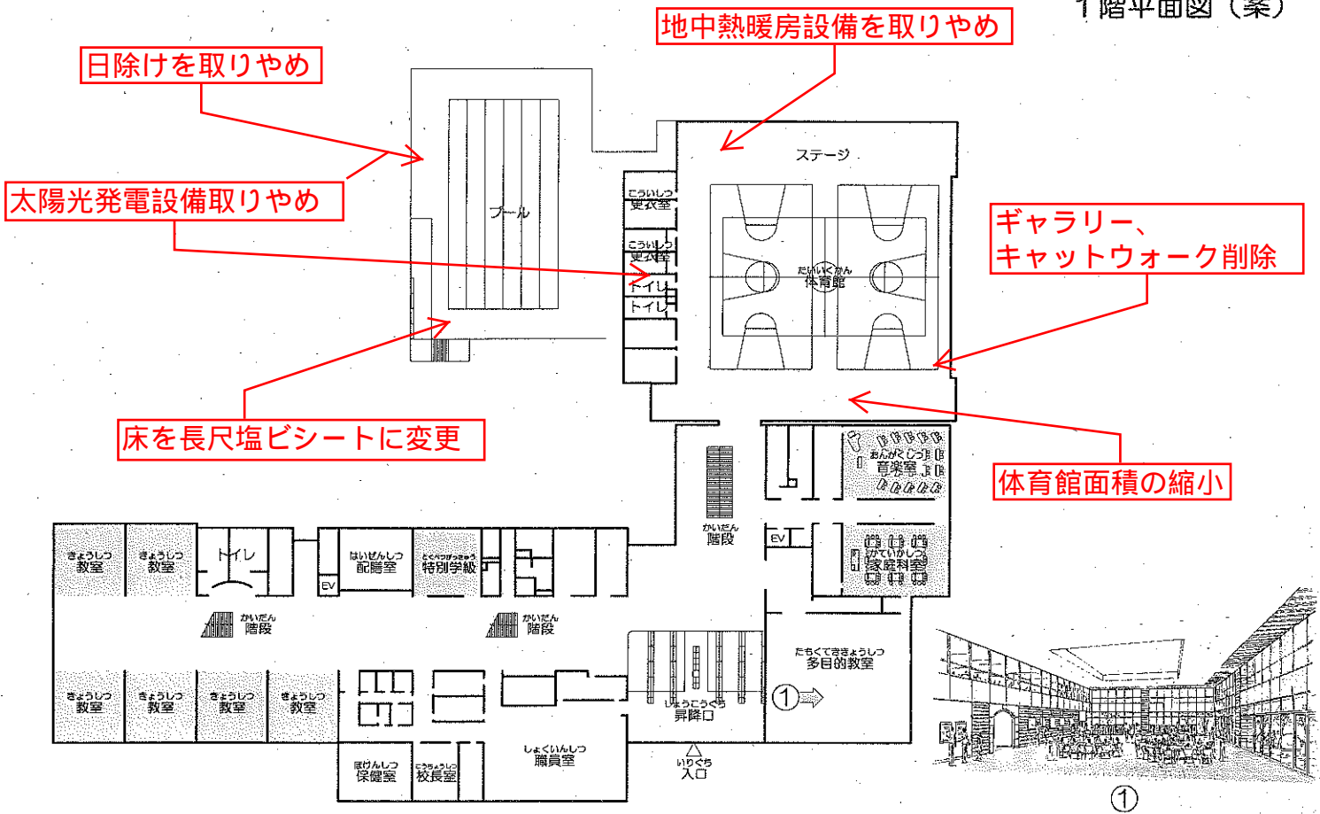
1階平面図 (案)
